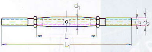
ASS Super-Mini-Ridoir à deux terminaisons simples
